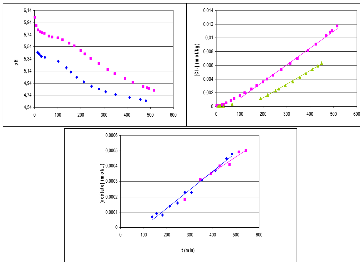
Figure 1: Suivi de la migration des ions H^+ , Cl^- et CH_3COO^- en fonction du temps à travers la viande, pour différentes solutions d'immersion : (♦) 0,1 mol.kg -1 d'acide acétique, (▲) 80 g.kg -1 de NaCl et (■) 0,1 mol.kg -1 d'acide acétique + 80 g.kg -1 de NaCl.
