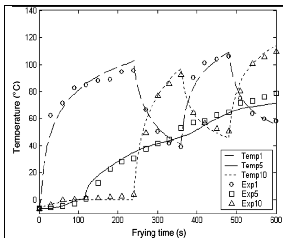
Figure 1 : Températures mesurées et simulées lors de la cuisson par simple contact d'un steak haché de 9.5 mm d'épaisseur sur une plaque portée à 160°C. Temp 5, 1 et 10 correspondent aux températures simulées respectivement au centre, et à proximité des 2 faces de l'échantillon. Les symboles correspondent aux mesures effectuées aux mêmes points (d'après Ou et Mittal, 2007).
