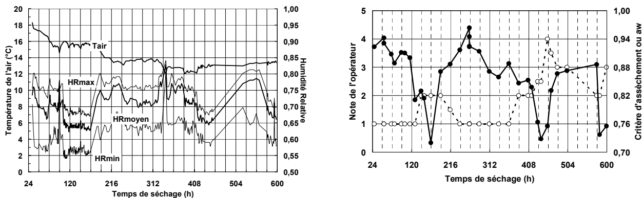
Figure 1 : (gauche) variation des conditions d'étuvage et de séchage imposées lors d'un essai mené avec le détecteur d'assèchement, (droite) note attribuée par l'opérateur sur une échelle 1 à 5 (o) et a_w moyenne estimée (●)
