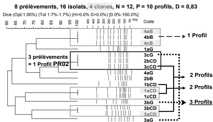
Figure 1 : Exemple d'analyse d'un dendrogramme obtenu après macrorestriction avec l'enzyme Sma 1 des souches de C. coli isolées à partir d'un lot. Code intra-lot = animal, isolat, nature du prélèvement (CD, B, G). Les 4 isolats considérés comme clones sont grisés.
